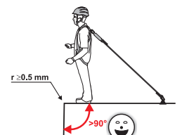
Certified for horizontal use over an edge Certificado para uso en horizontal sobre bordes
